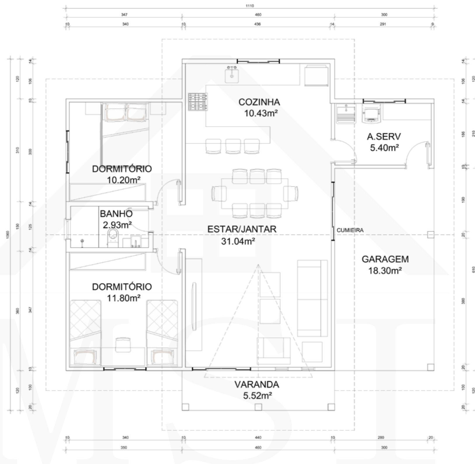
CASA _ PLANTA BAIXA ÁREA TOTAL=102,05m 2
