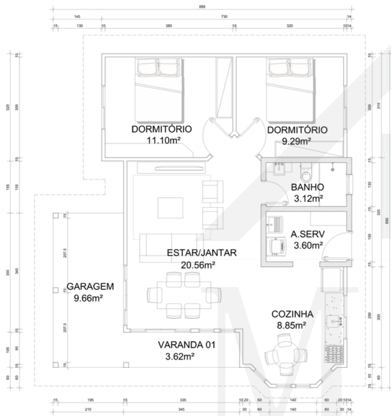
CASA_PLANTA BAIXA ÁREA TOTAL=75,57m²
