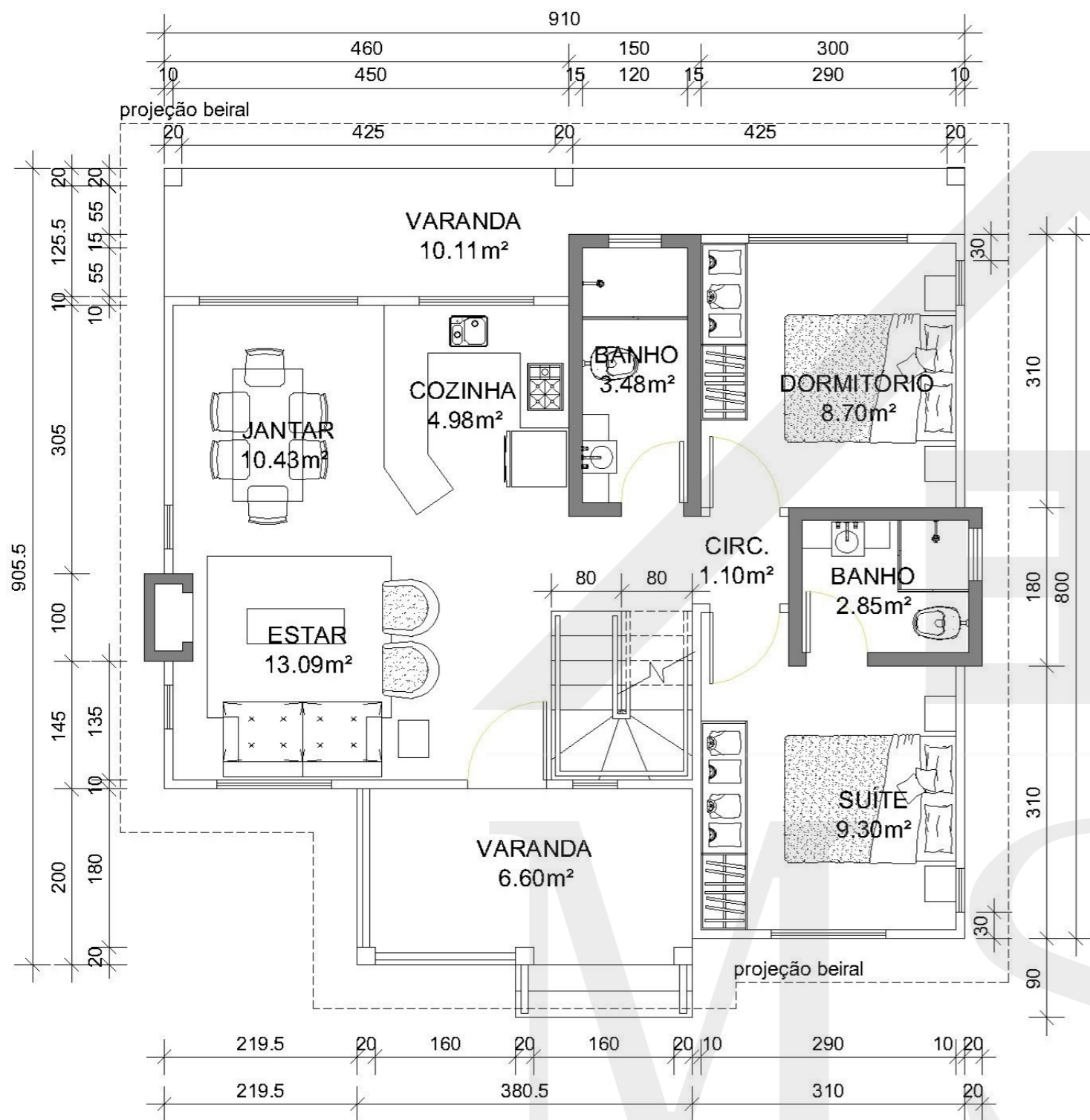
PLANTA BAIXA PAV. TÉRREO
